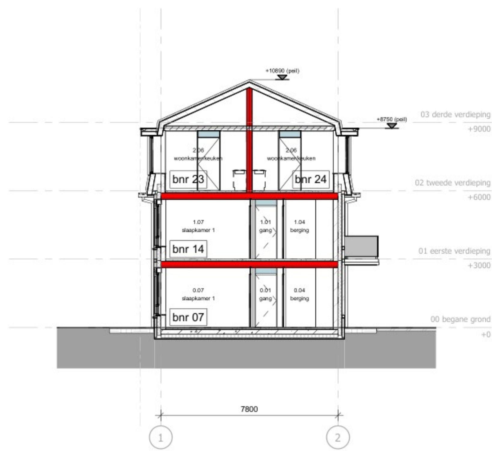
doorsnede C-C
