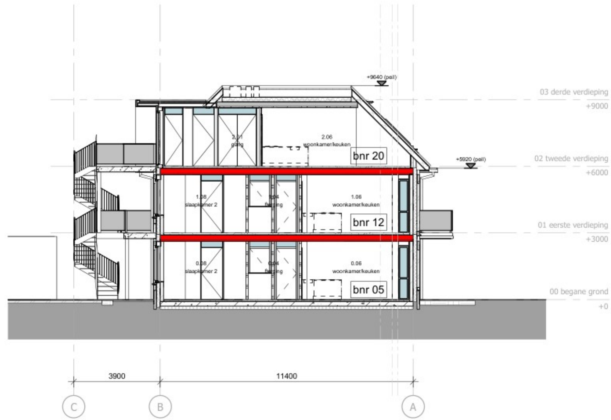
doorsnede B-B
